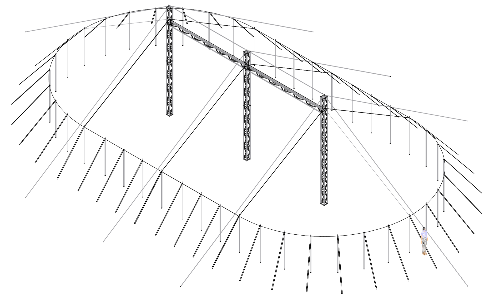
3 Pole 24.3 x 12.2 Meter
