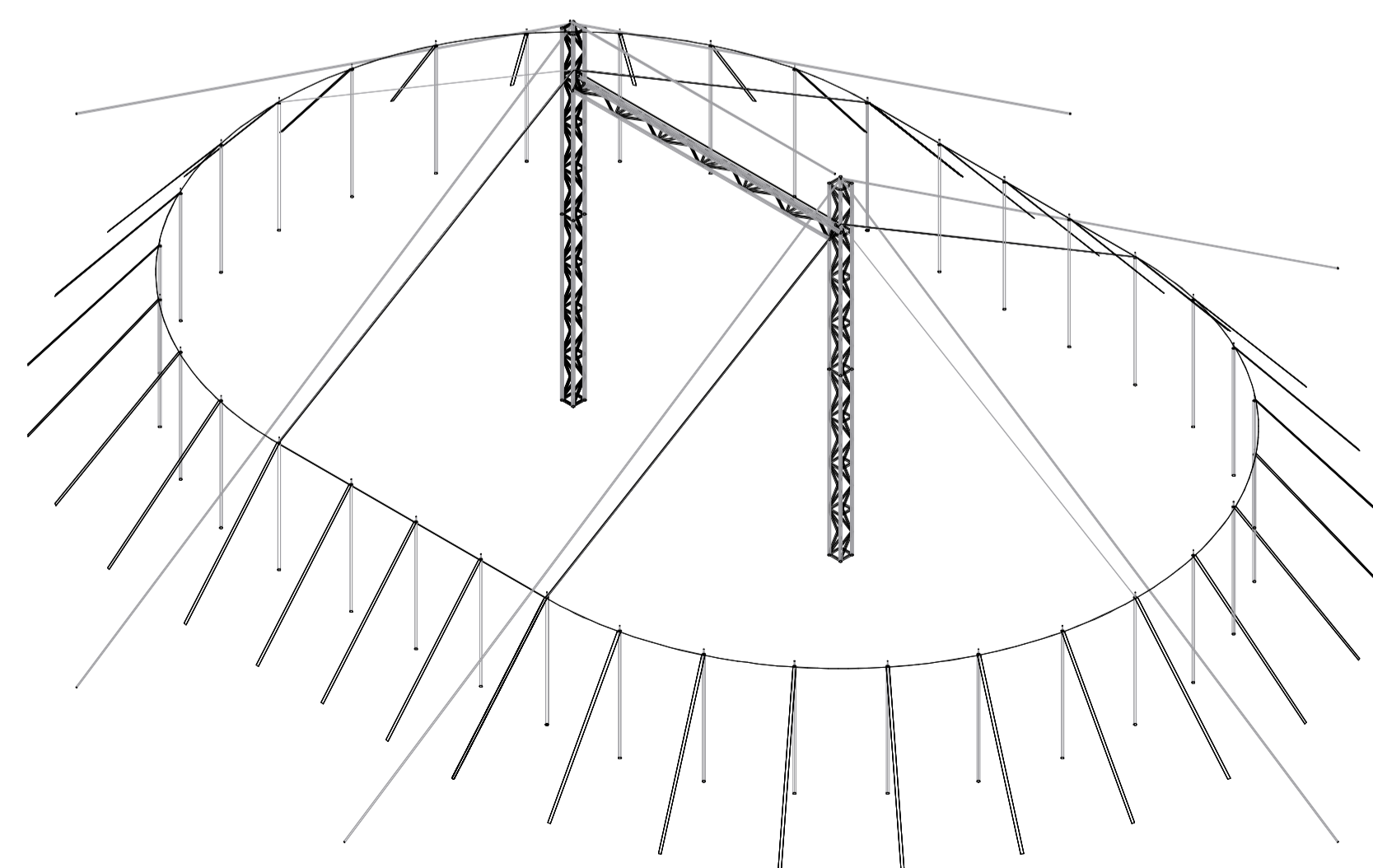
2 Pole 18.5 x 12.2 Meter
